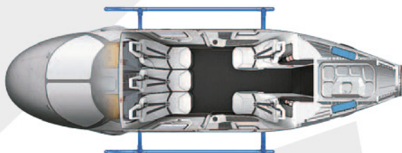
Компоновка VIP-салона
