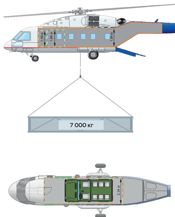
Компоновка транспортного варианта
