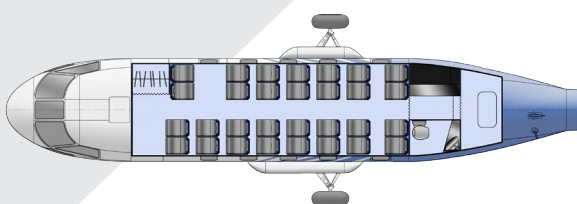
Компоновка пассажирского варианта на 30 мест
